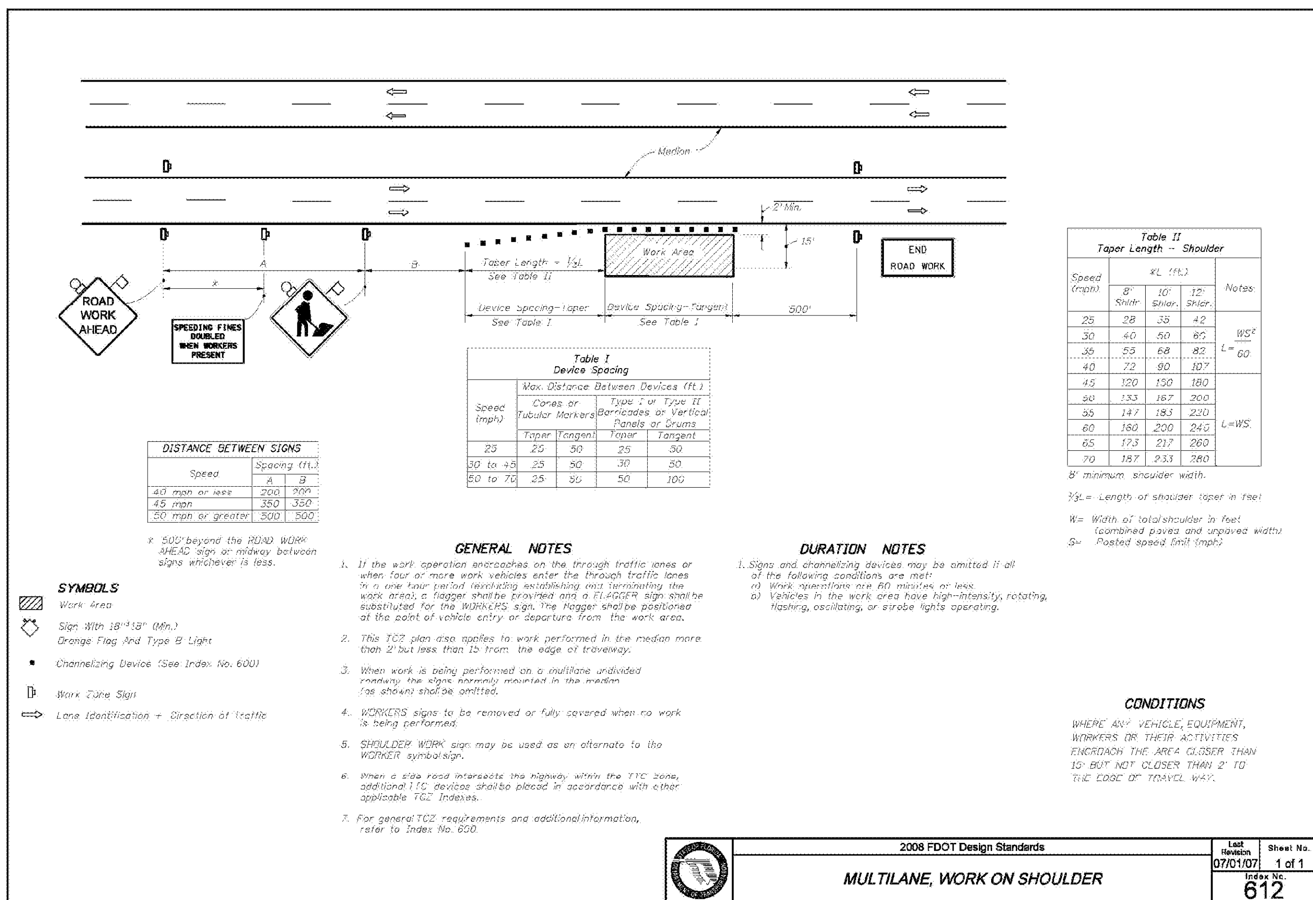
FDOT INDEX 612
