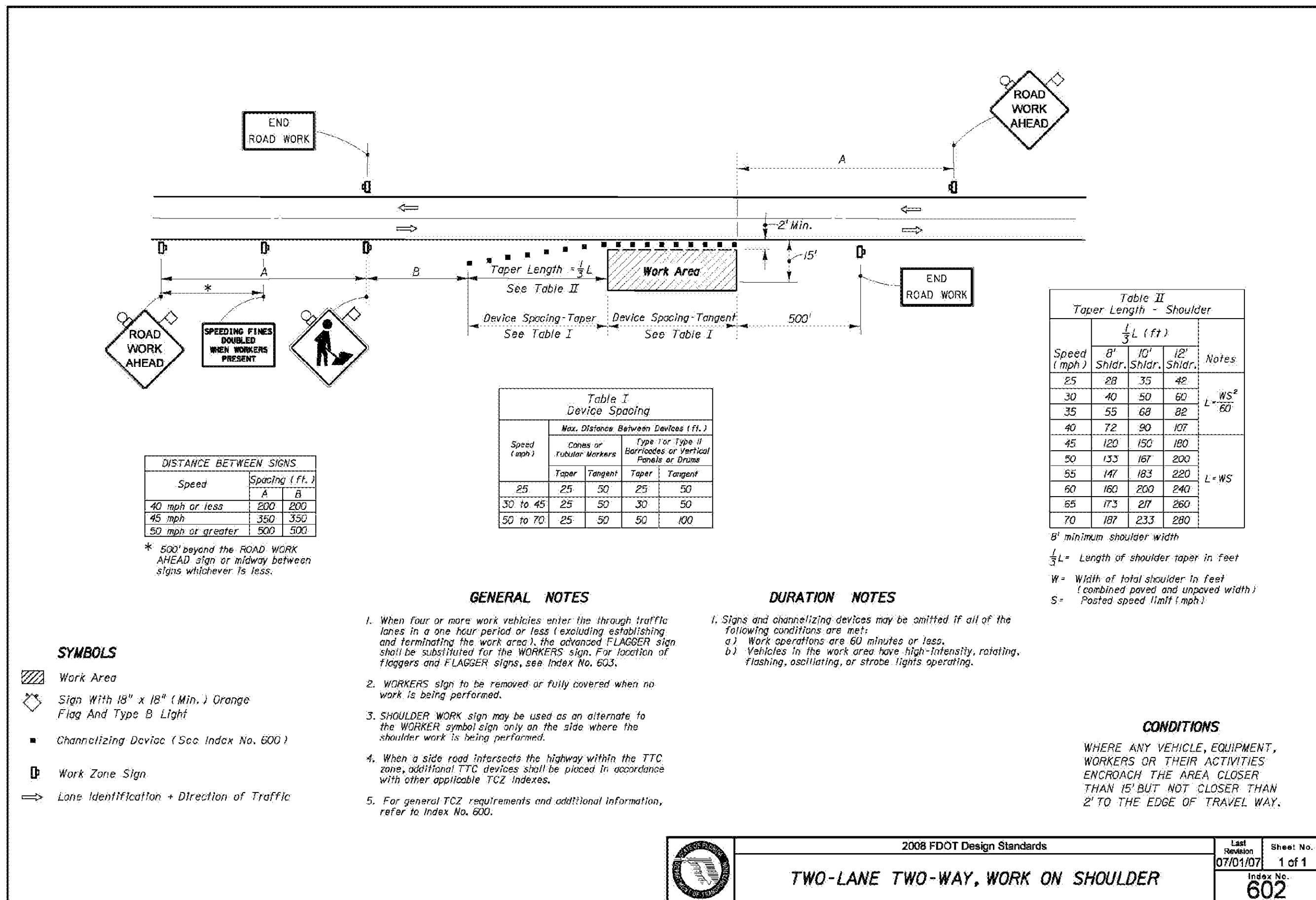
FDOT INDEX 602
