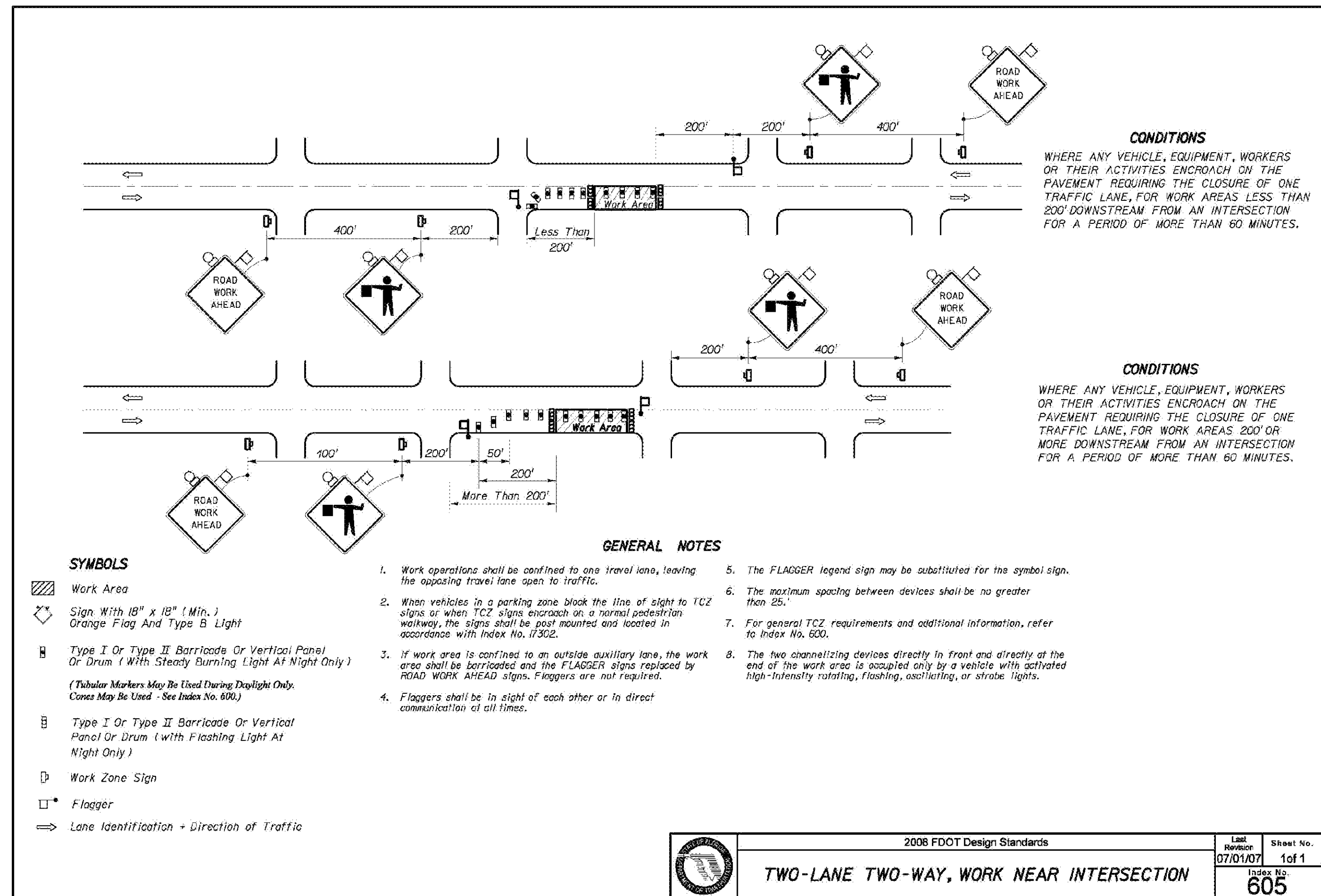
FDOT INDEX 605
