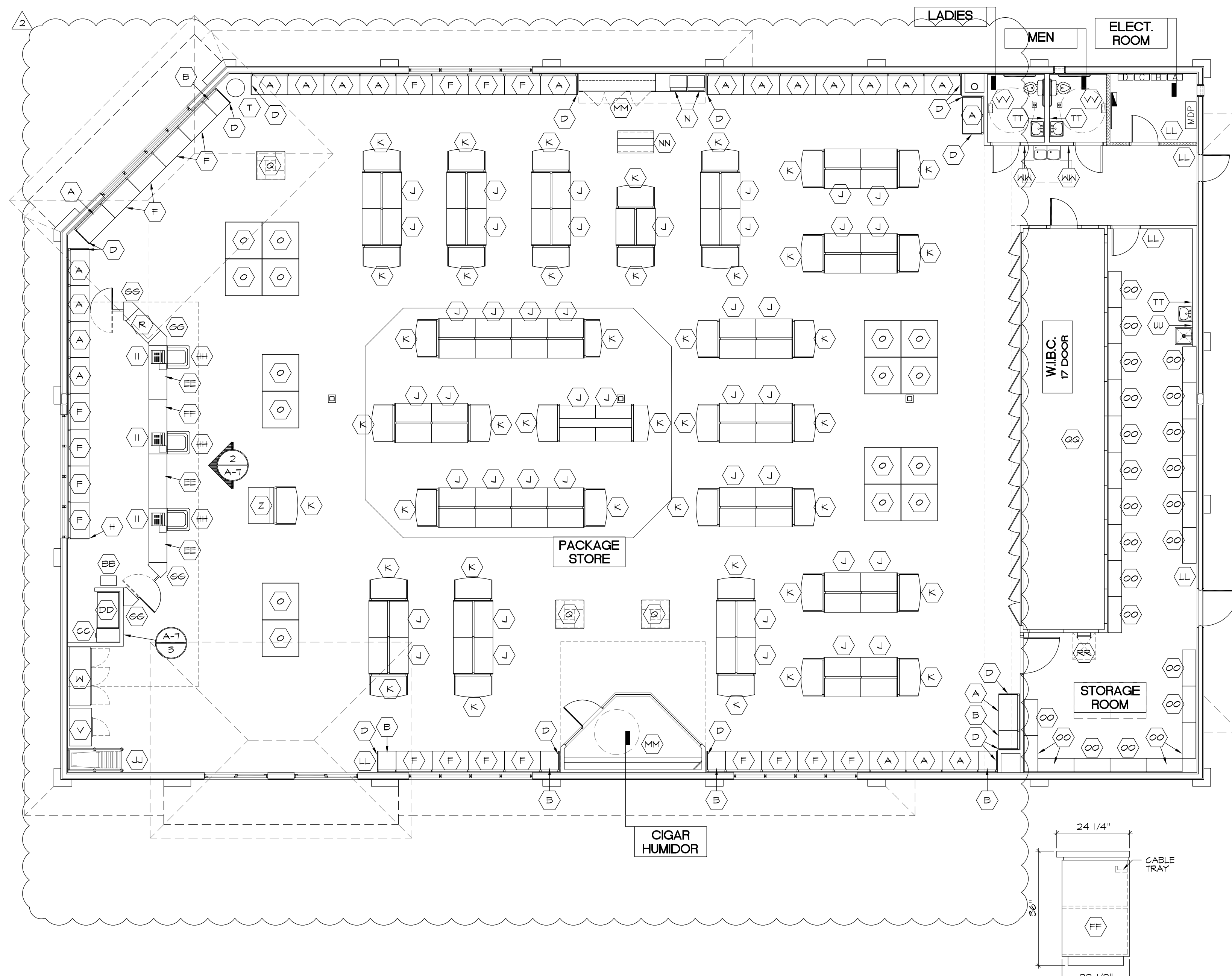
1 #197 FURNITURE PLAN SCALE: 1/8" = 1'-0"
