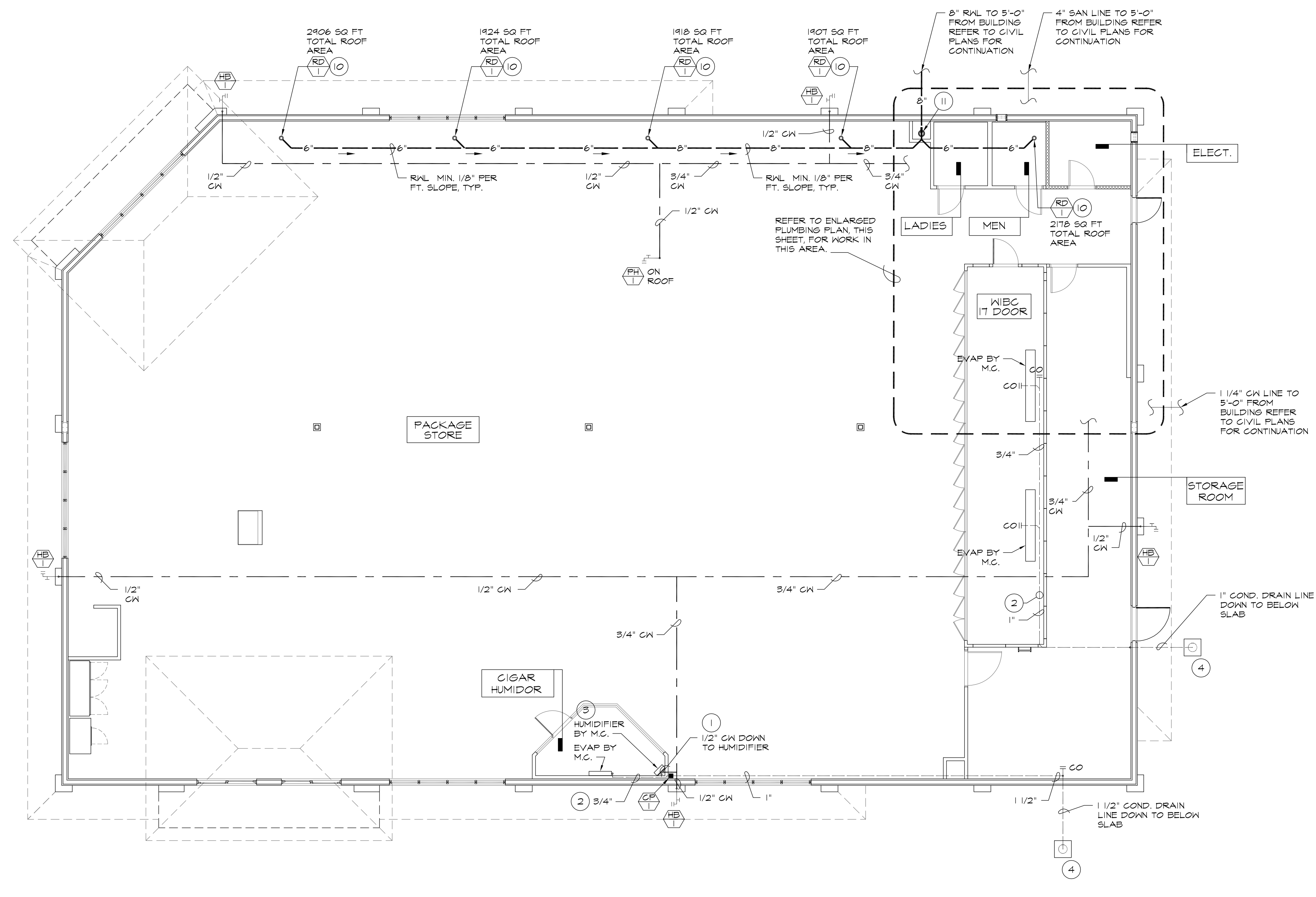
1 PLUMBING PLAN SCALE: 1/8" = 1'-0"
