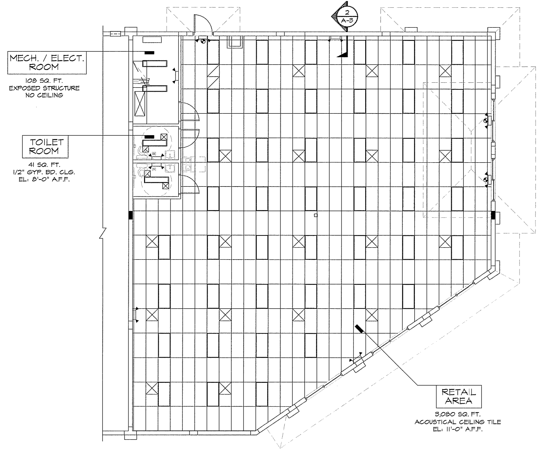
1 REFLECTED CEILING PLAN A-3 SCALE: 1/8" = 1'-0"
