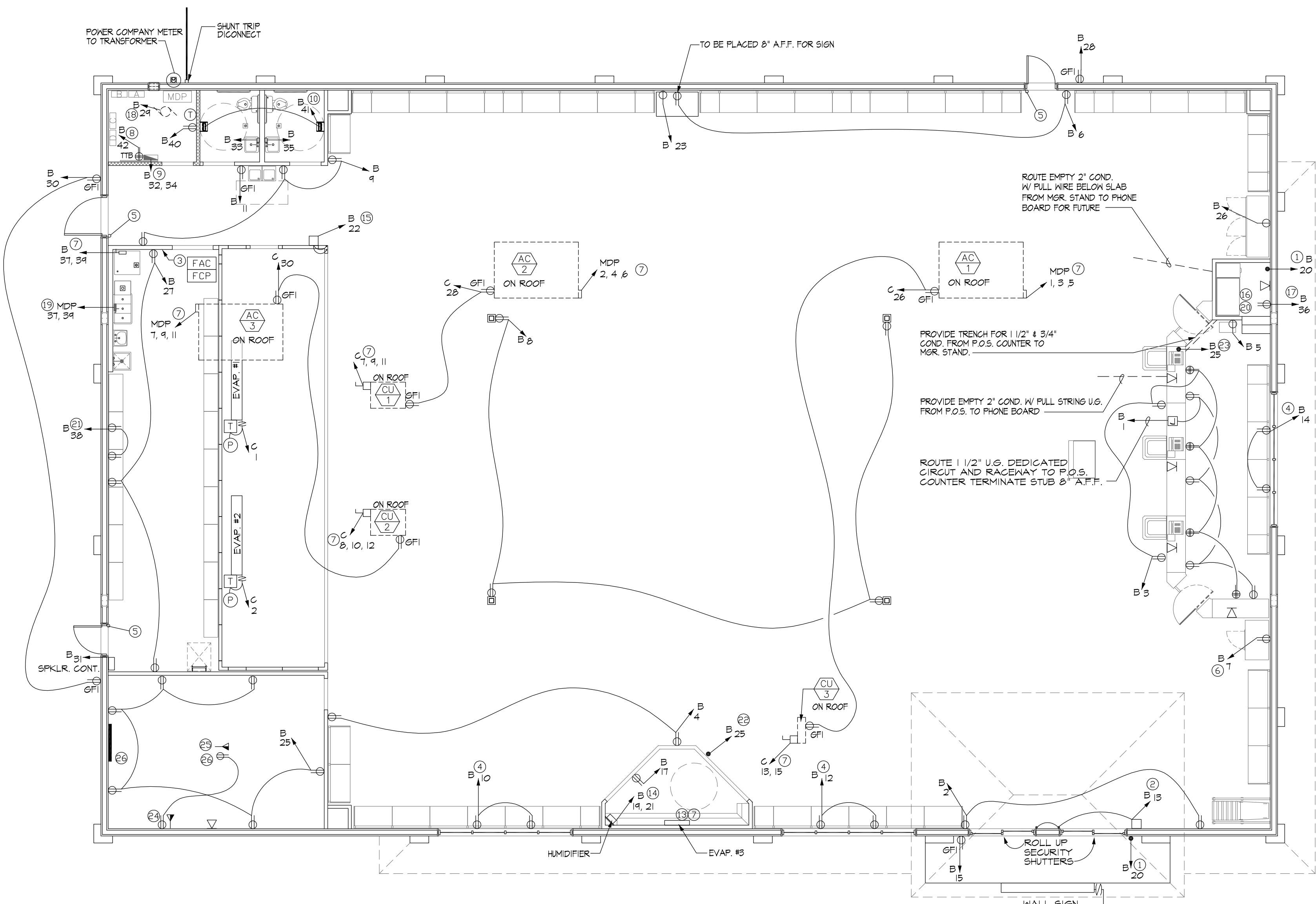
1 POWER PLAN E-3 SCALE: 1/8" = 1'-0" TRUE PROJECT
