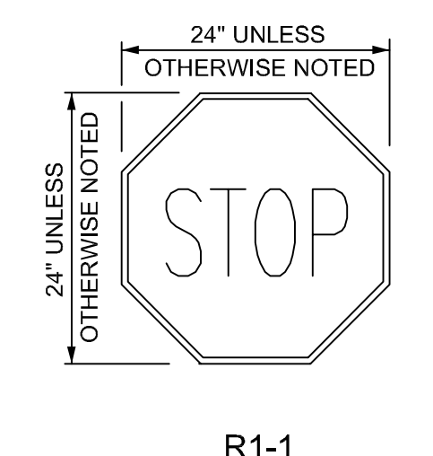
R1-1 M.U.T.C.D. SIGN DETAILS N.T.S.
