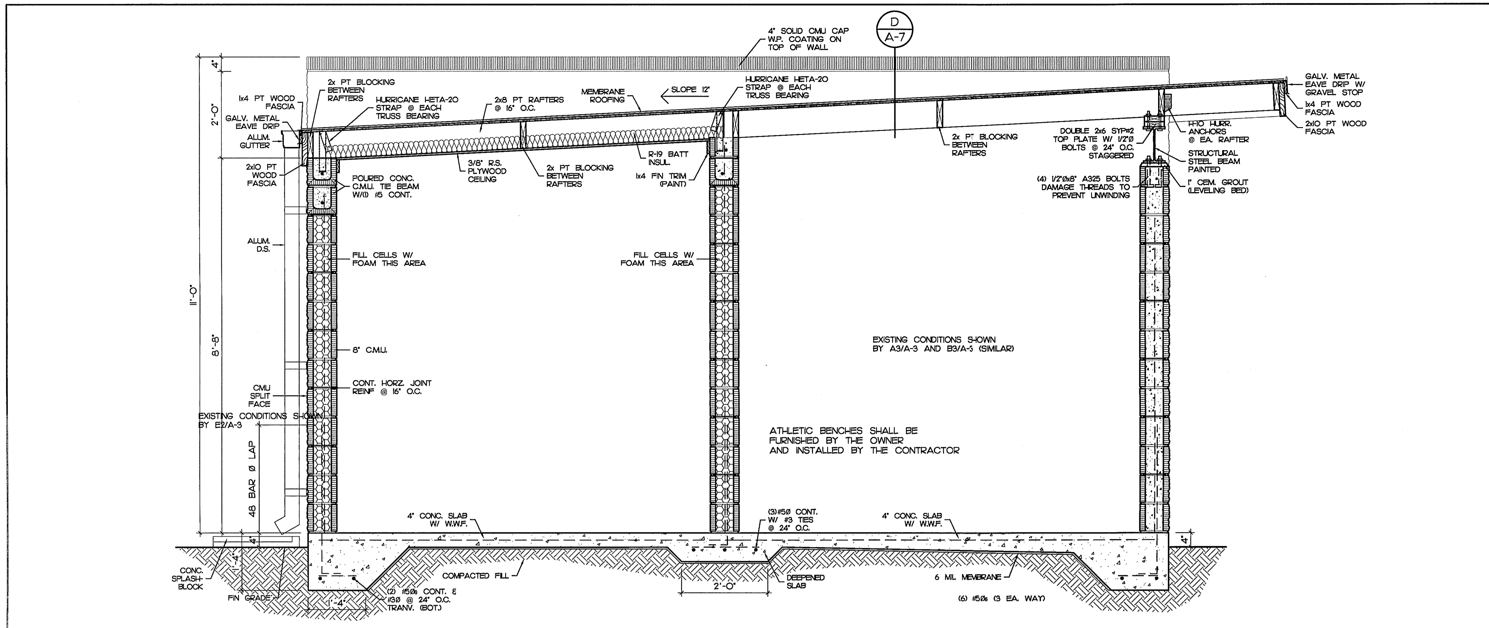
A SECTION SCALE: 3/4" = 1'-0"
