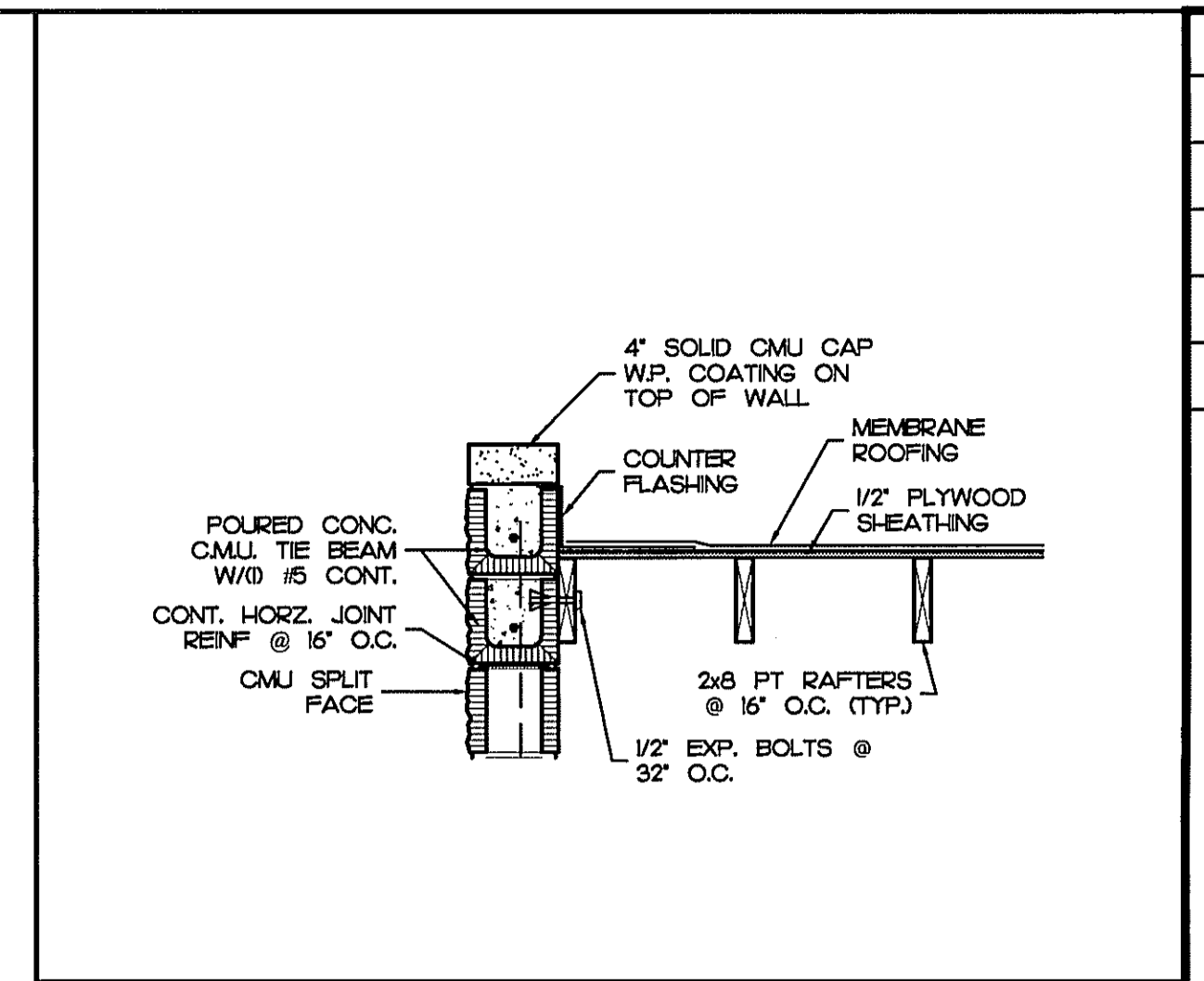
D DETAIL SCALE: 3/4" = 1'-0"
