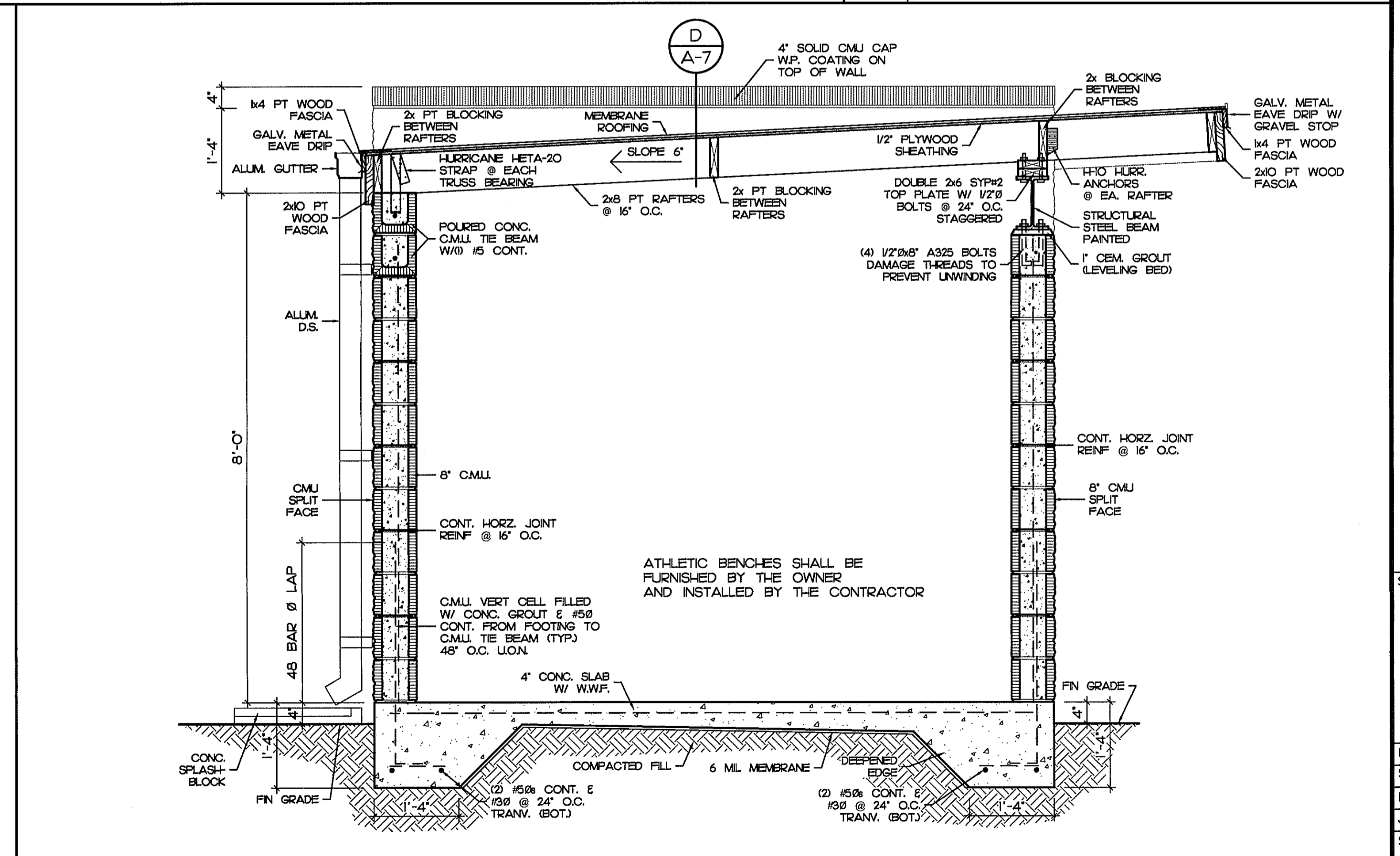
C SECTION SCALE: 3/4" = 1'-0"
