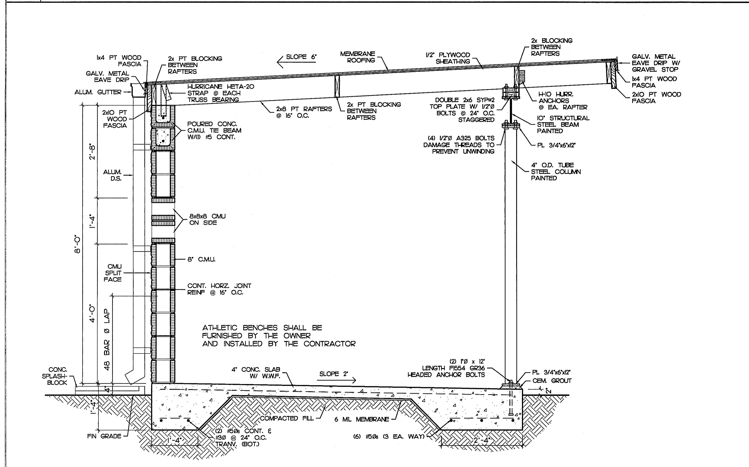
B SECTION SCALE: 3/4" = 1'-0"
