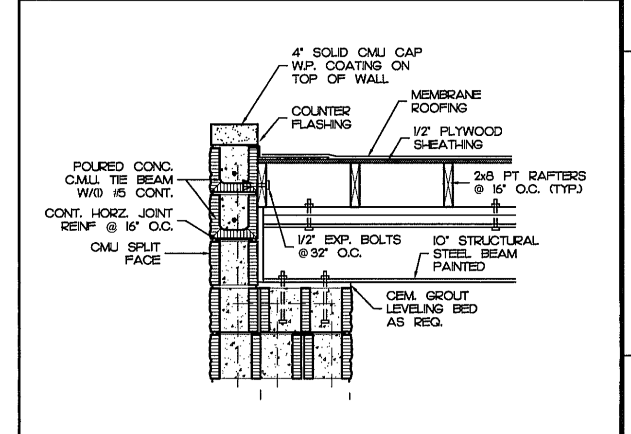
E DETAIL SCALE: 3/4" = 1'-0"
